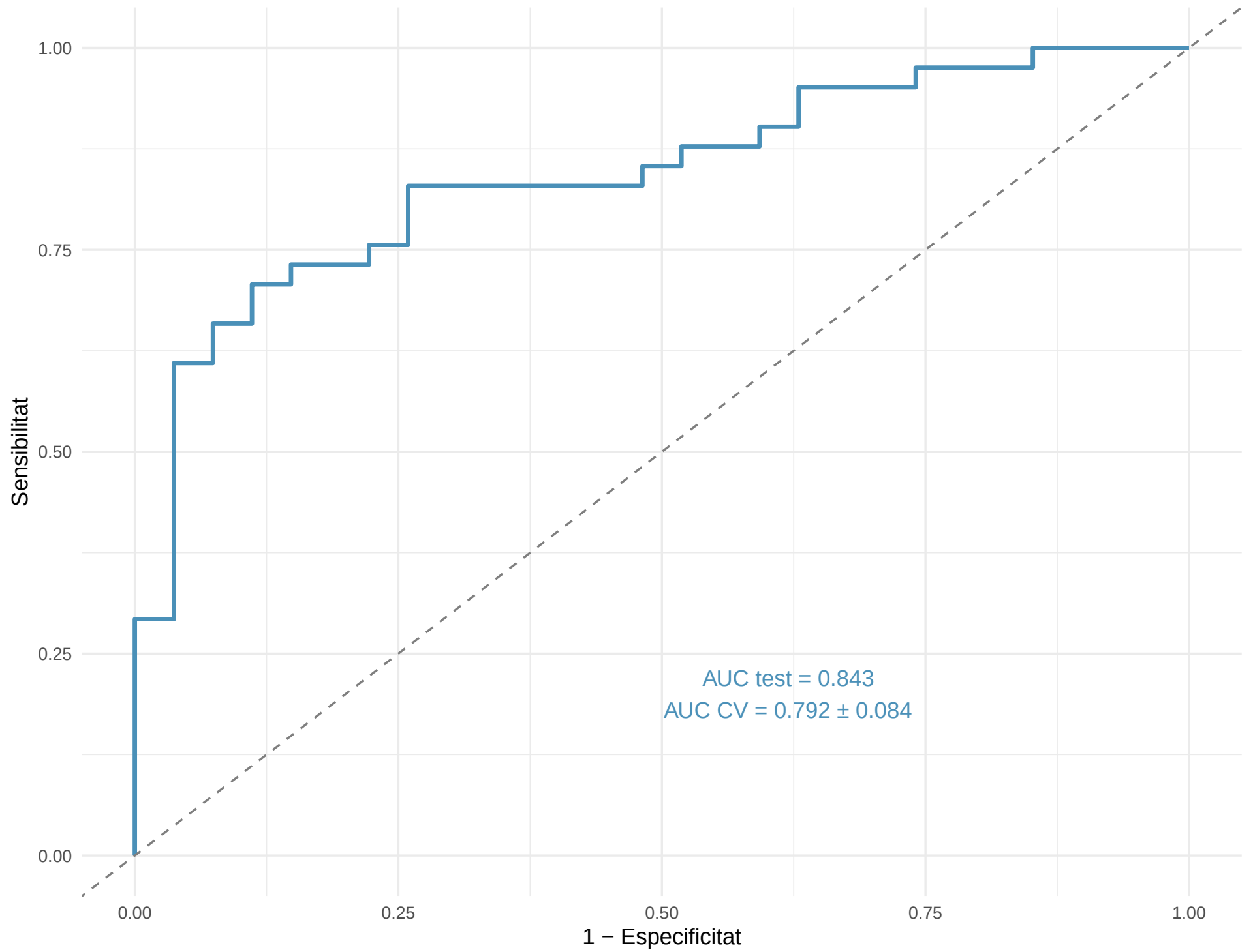
Corba ROC — Model logístic (test)
